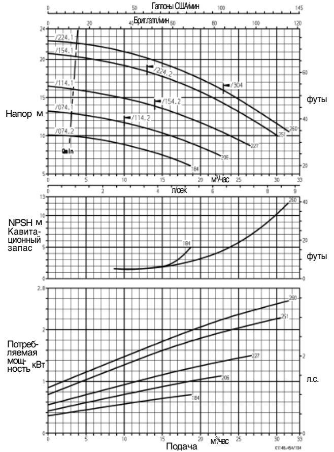
Etaline Z 40-250
